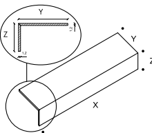
Elemento a L personalizzabile Service | su richiesta
